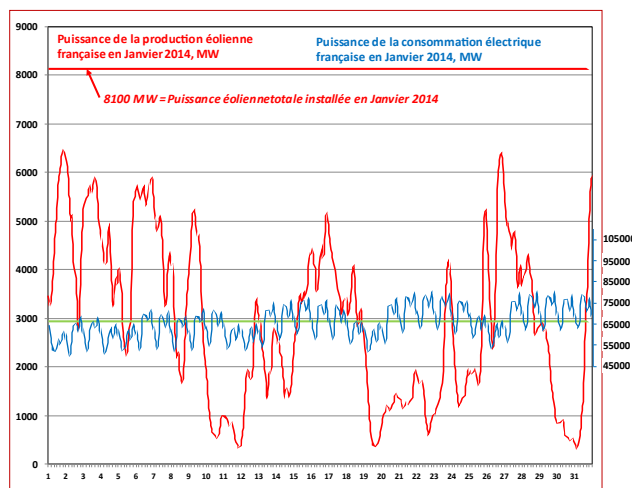
FIGURE 7 : PUISSANCE ÉOLIENNE ET CONSOMMATION D'ÉLECTRICITÉ EN FRANCE :
