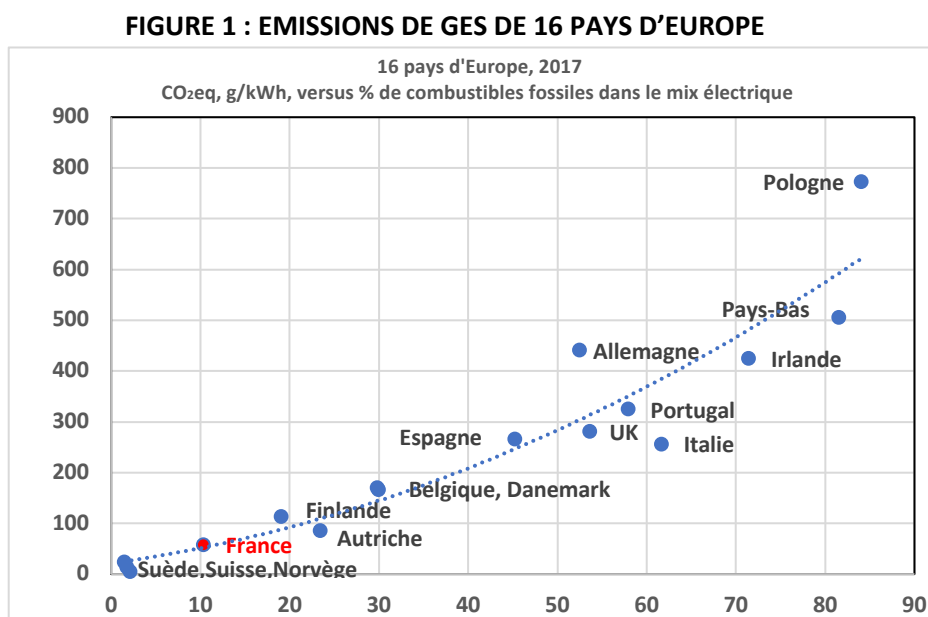
Figure 1: Emissions de CO 2 eq du mix de production électrique 2017 de 16 pays d'Europe de l'Ouest en fonction du % des combustibles fossiles dans ce mix. Les valeurs plus fortes d'émissions de CO 2 eq pour une même proportion de combustibles fossiles viennent essentiellement de la nature des combustibles utilisés, charbon plutôt que gaz. Source des données :Eurostat et Agence européenne de l'environnement.
