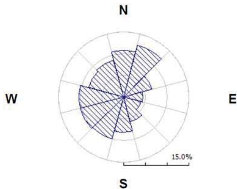
Rose des vents à long terme
