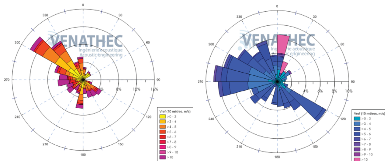
Rose des vents pendant la campagne de mesure
