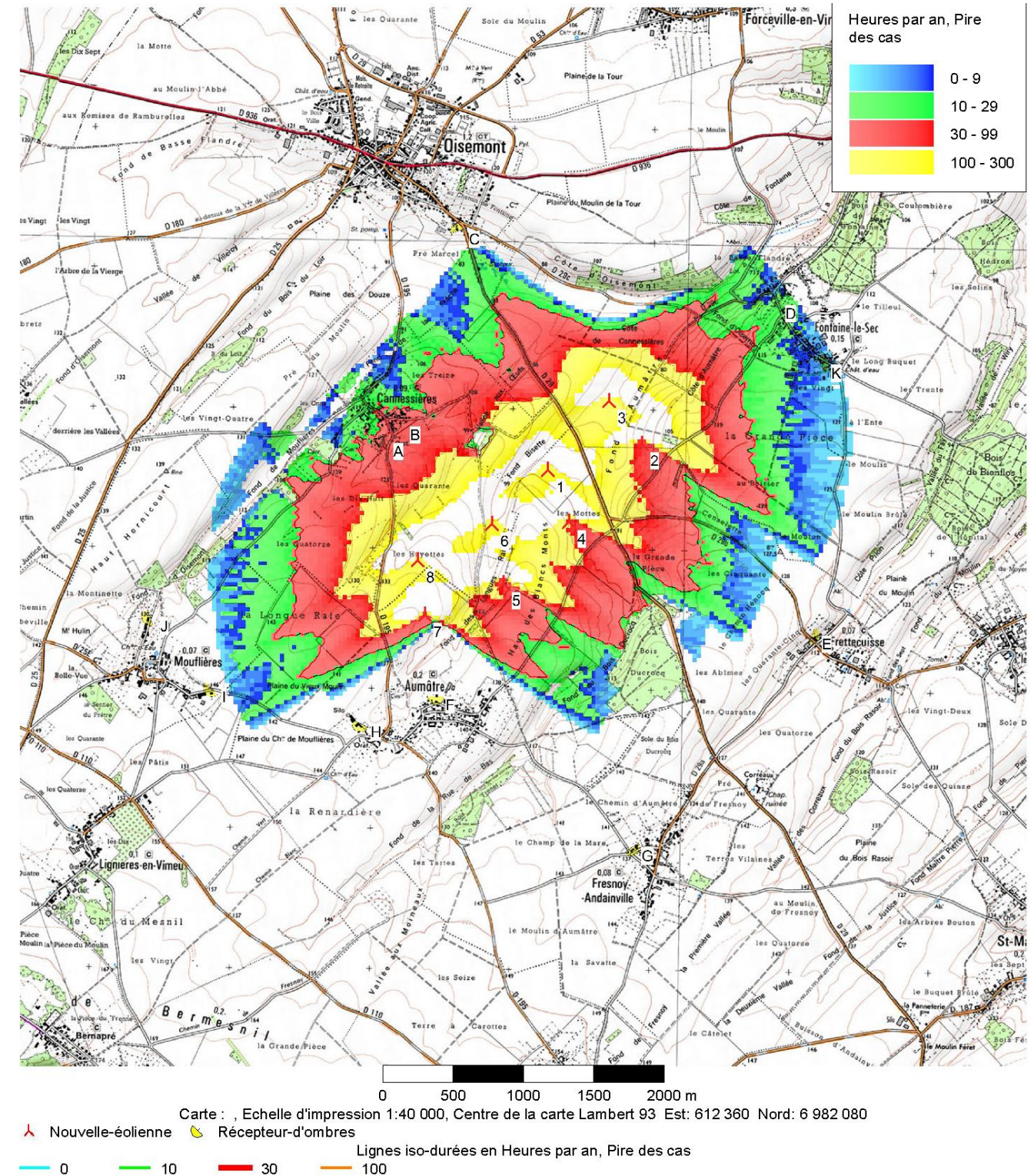
Carte 7 : Zones d'exposition aux ombres
