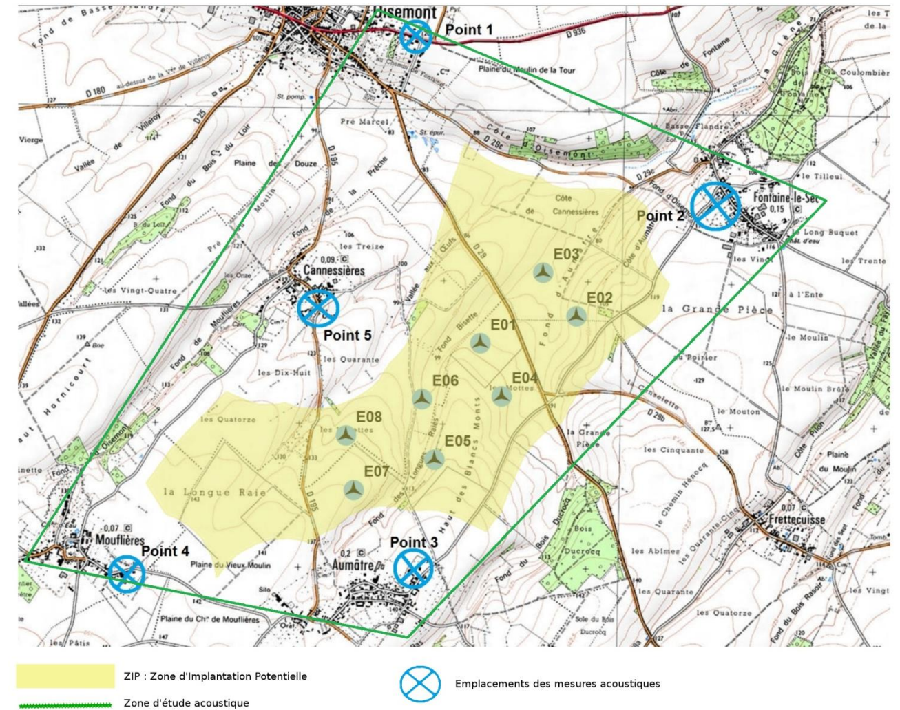
Carte 6 : Localisation des points de mesure acoustique (Source – KIETUDES)
